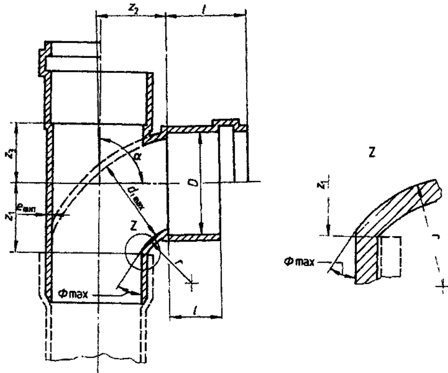
Рисунок Г.4 – Відгалуження крутозагнуте (87\frac{1}{2} - 88\frac{1}{2})^\circ з гладким кінцем
