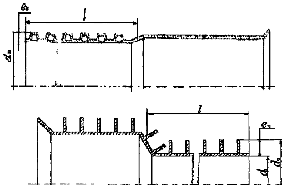
Рисунок 4 – Будівельна довжина труб розтрубних типу В
