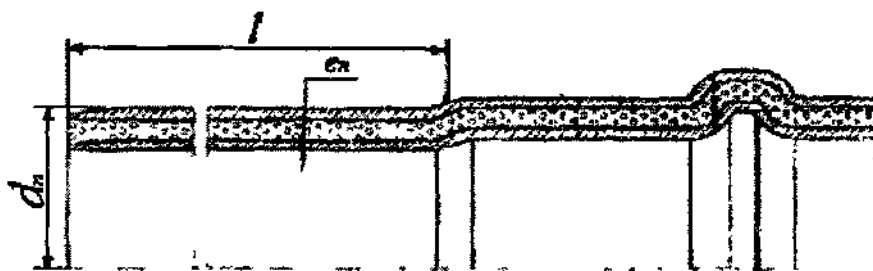
Рисунок 3 – Будівельна довжина труб розтрубних типу А
