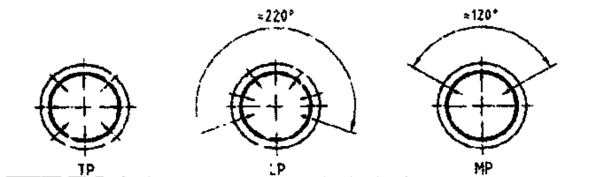
Рисунок Б.1 – Основні типи труб дренажних в залежності від розміщення перфорації.
