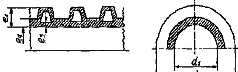
Рисунок 8 – Повздовжній і поперечний перерізи труб типу В (без розтруба) в конструктивному виконанні з гофрованою поверхнею та гладкої частини труб розтрубних типу В
