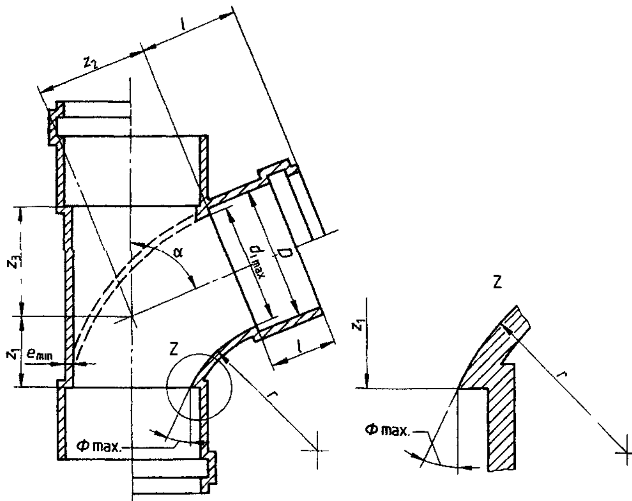
Рисунок Г.7 – Відгалуження крутозагнуте 67\frac{1}{2}^\circ
