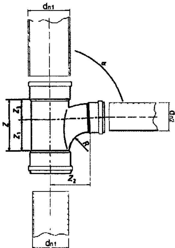
Рисунок 17 – Відгалуження крутозагнуте
