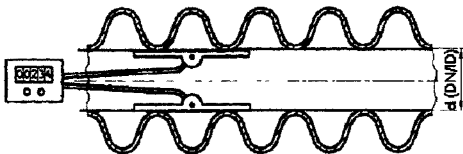
Рисунок 34 – Приклад використання вимірювального обладнання з цифровим індикатором
