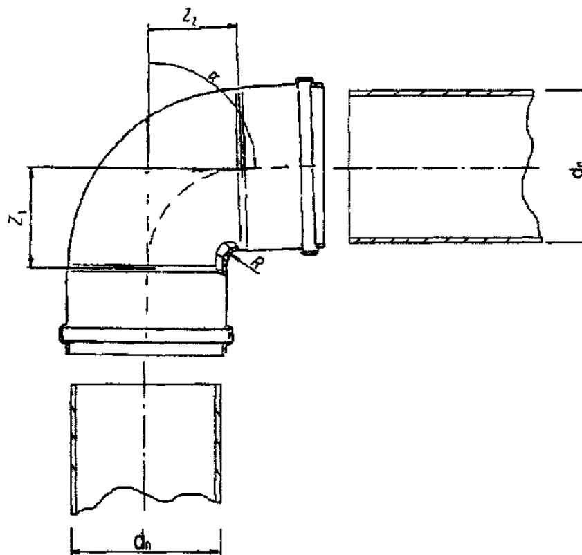
Рисунок 13 – Коліно
