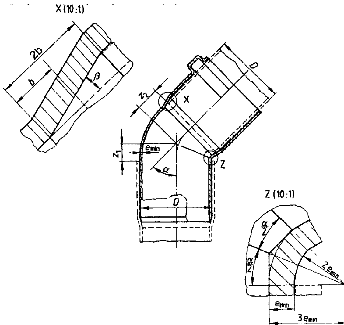
Рисунок К.1 – Коліно з гладким кінцем
