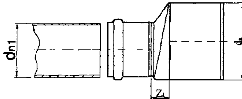
Рисунок 19 – Перехід
