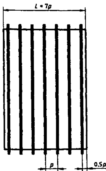
Рисунок 33 – Приклад зразка для визначення кільцевої жорсткості труб типу В
