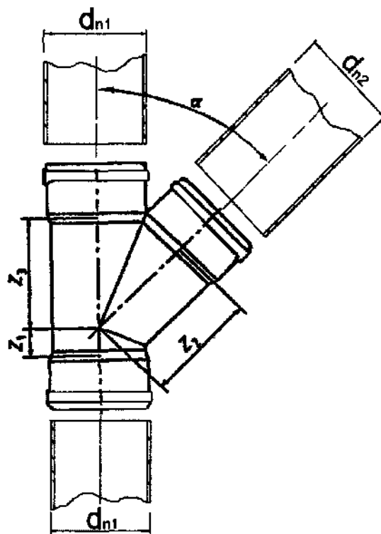
Рисунок 15 – Відгалуження
